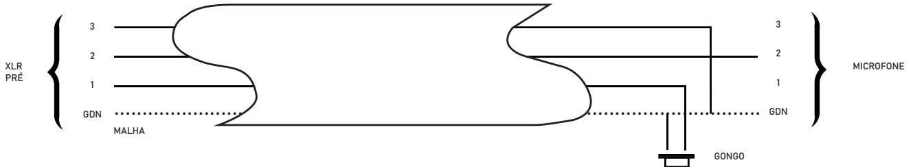
MICROFONE DESBALANCEADO
