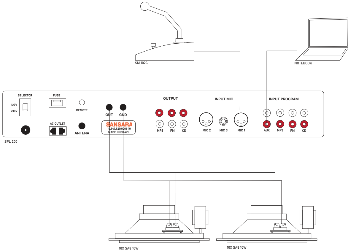
MICROFONE BALANCEADO
