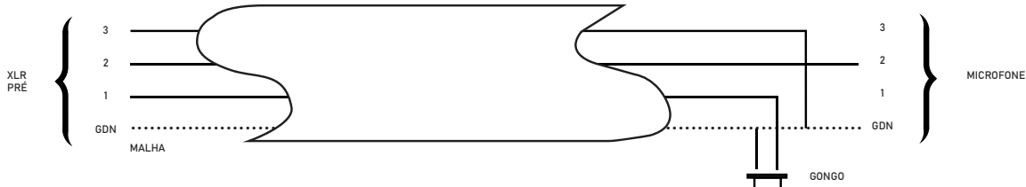
MICROFONE DESBALANCEADO
