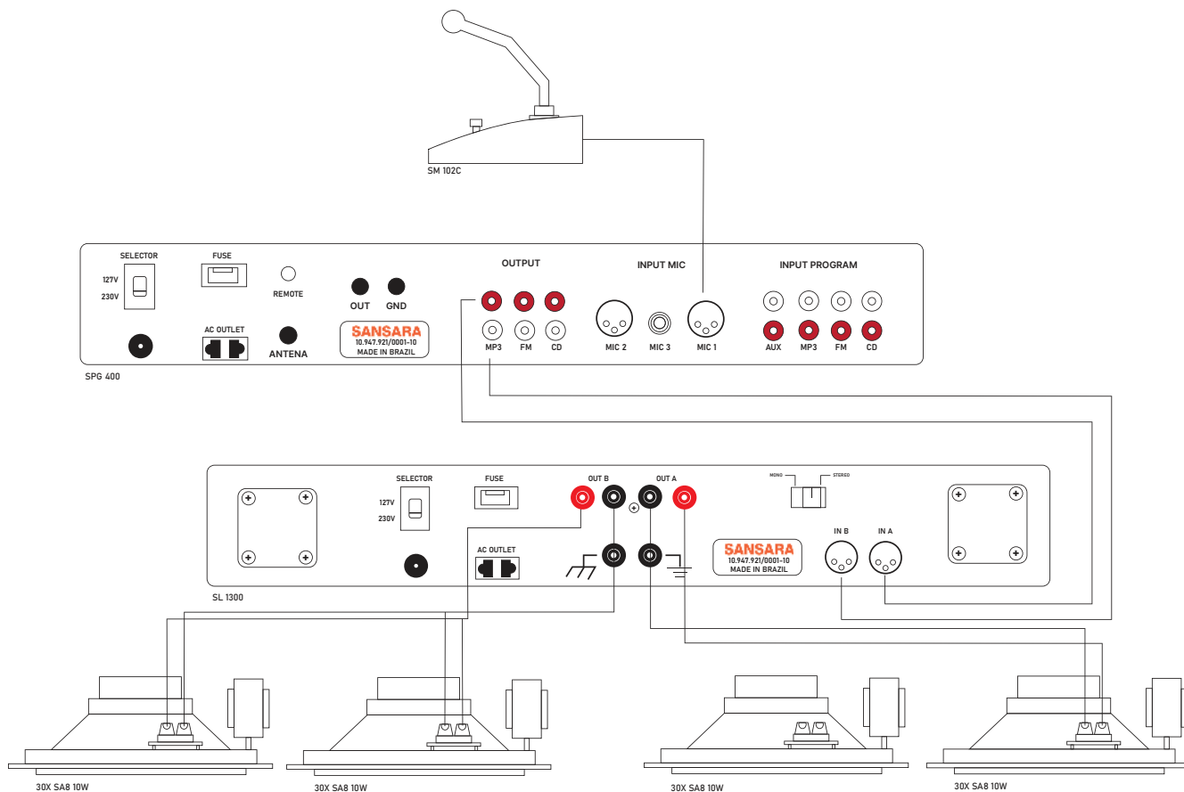
MICROFONE BALANCEADO
