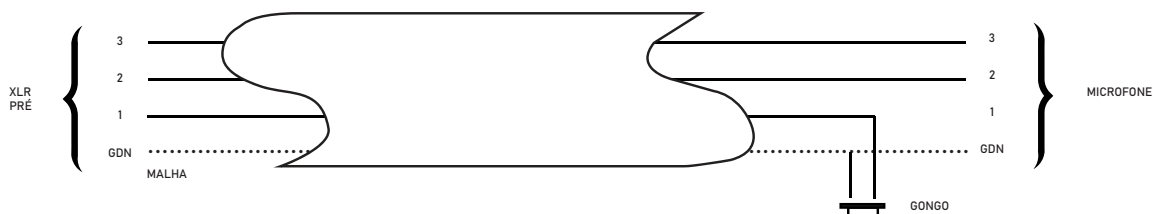
MICROFONE DESBALANCEADO
